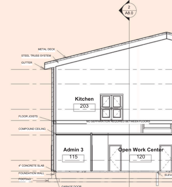
1 Longitudinal Section 1/8" = 1'-0"
